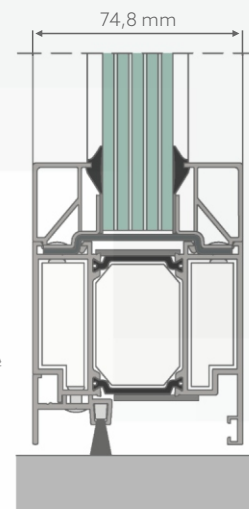
PRZEKRÓJ PRZEZ DRZWI ZE SZCZOTKĄ
