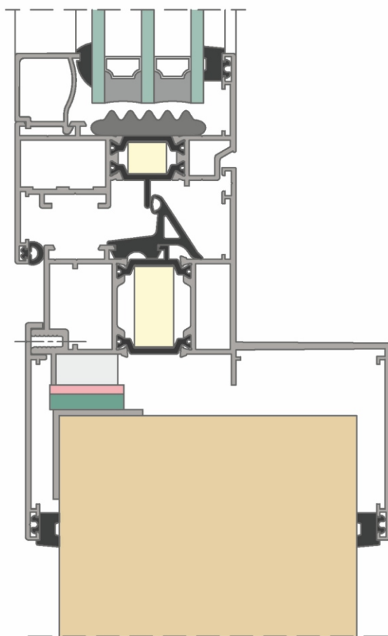
OKNO W PŁYCE WARSTWOWEJ
